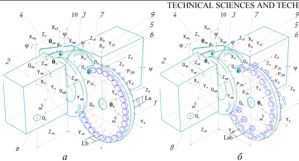
Рис. 1. Розрахункова схема формоутворення торців деталей різних діаметрів з двома способами розташування їх у барабані подачі
