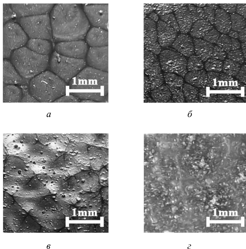
Рис. 6. Макроструктура поверхні композиційних покриттів на основі фенілоноу, що містять 30 мас.% наповнювача: а – дисульфід молібдену; б – графіт; в – фталоціанін міді; г – нітрид бору
