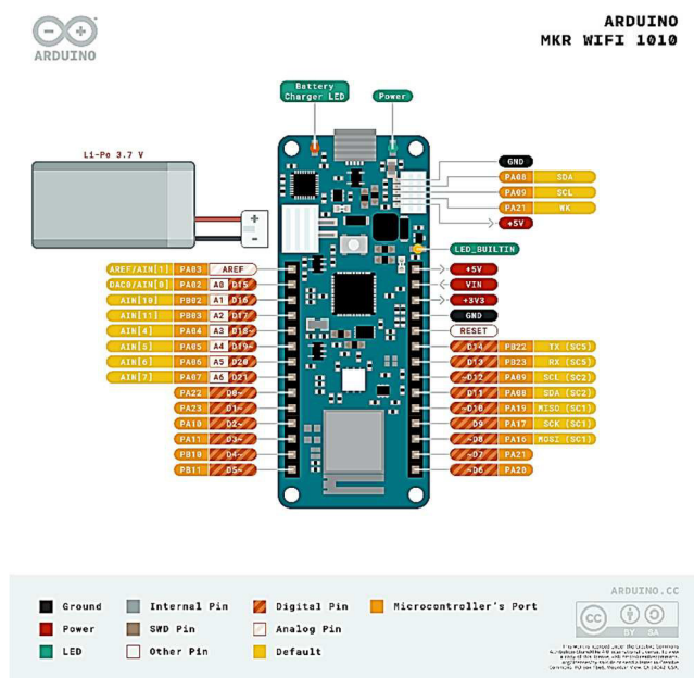
Fig. 7. Arduino MKR 1010 [11]
