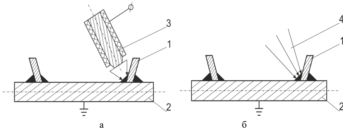
Рис. 2. Приєднання утримувача до робочої пластини за допомогою електродугового зварювання плавким електродом (а) або лазерного випромінювання (б) [2; 3; 4; 5]
