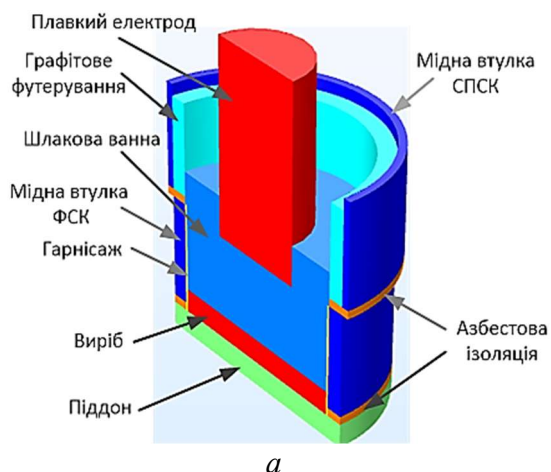
Рис. 3. Мультифізична модель стаціонарного СПК з плавким електродом: а – структура СПК; б – розрахункова сітка СПК
