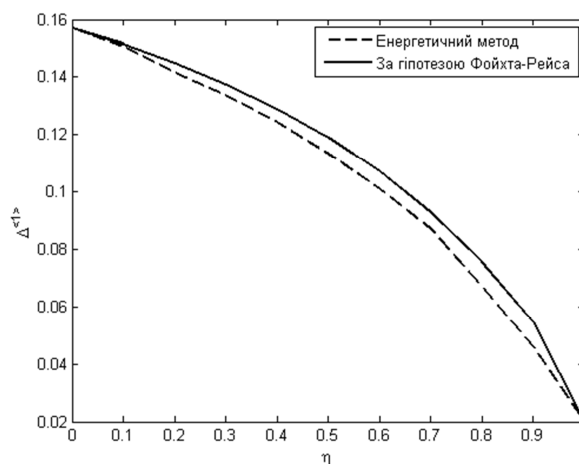
Рис. 4. Залежність декременту коливань від коефіцієнта армування двокомпонентного матеріалу за двома методами
