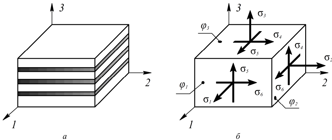
Рис. 1. Елемент об'єму багат шарової структури (а), напружений стан (б); ( \sigma_1 \dots \sigma_6 – напруження, \phi_1 \dots \phi_3 – електричні потенціали еквіпотенціальних граней одиничного об'єму)
