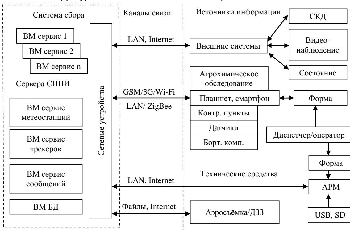
Рис. 4. Структурная схема ССПИ
