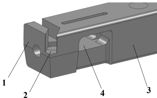
Рис. 6. Конструкция приспособления для трехкоординатного измерения усилия резания Резец-Т
