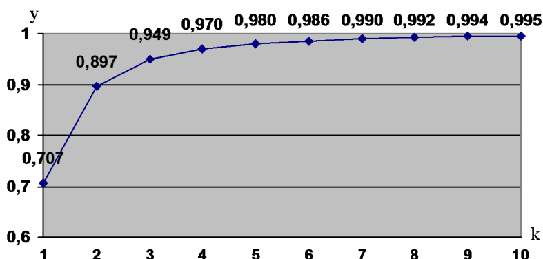
Рис. 2. Графік залежності y = k / \sqrt{k^2 + 1}
