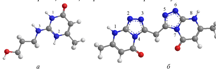
Просторові моделі (а - Ін 1; б - Ін 2) та розподіл зарядів на основних адсорбційно-реакційних центрах похідних піримідину
