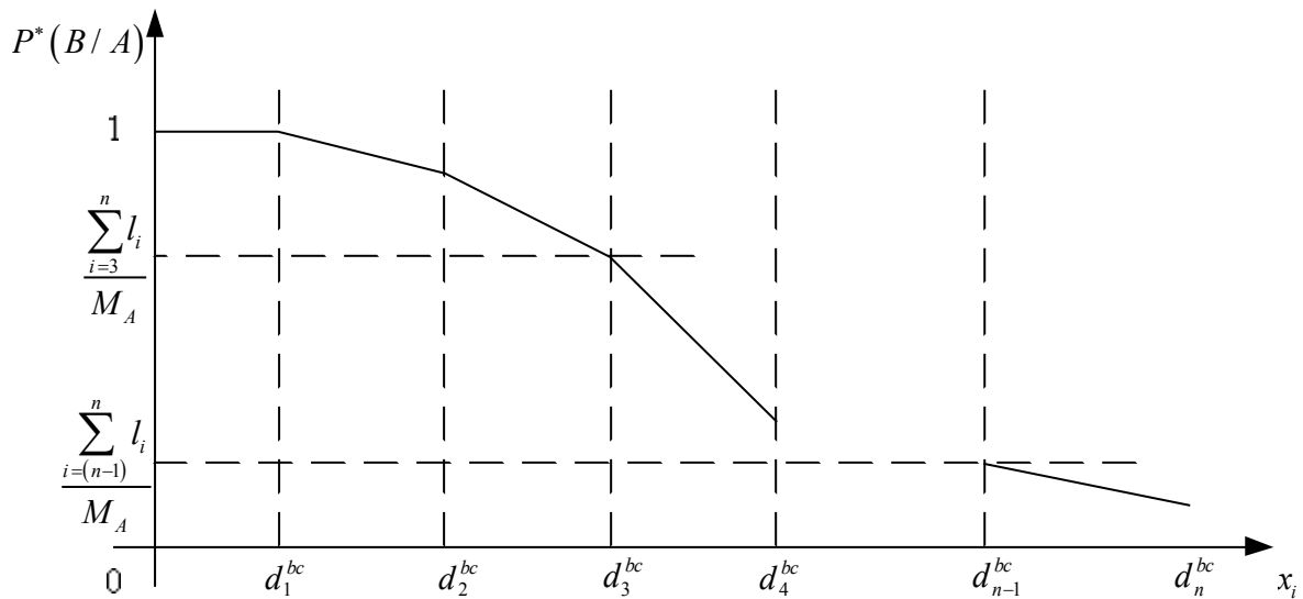
Рис. 2. Лінія регресії закону розподілу P^*(B\{d \leq d^{bc}\} / A) = f(x_i)
