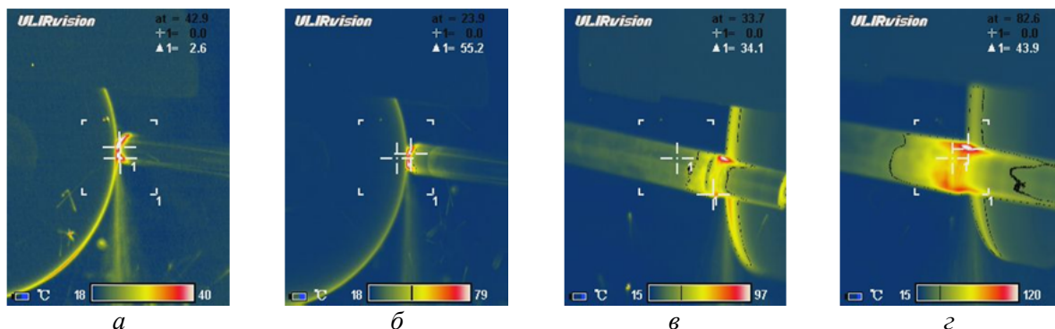
Рис. 4. Температури шліфувального круга і деталі у процесі глибинного однопрхідного шліфування при кутах схрещування осей 0,5° (а, б) та 1° (в, з)
