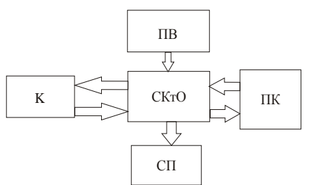
Рис. 6. Функціональна схема стенду
