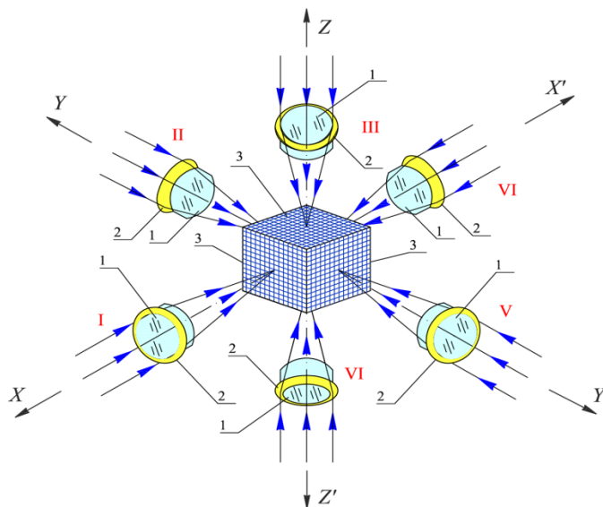
Рис. 4. Схема шестиканального оптико-електронного приладу-ДМ: 1 – об’єктиви цифрових камер; 2 – світлові елементи кільцевих джерел світла (візирна марка); 3 – багатоелементні фотоприймачі (матриці)
