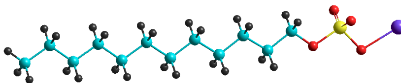
Рис. 1. Структура молекули SLS після оптимізації її геометрії (Nuper Chem 7.0, RHF розрахунок за методом MNDO-PM3)
