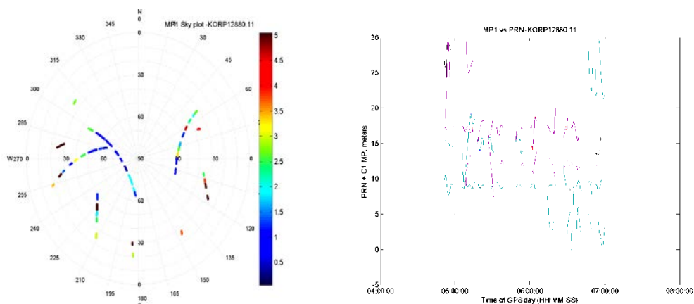
Рис. 1. Багатопроменевість та рисунок неба на частоті L1 для пункту KORP1
