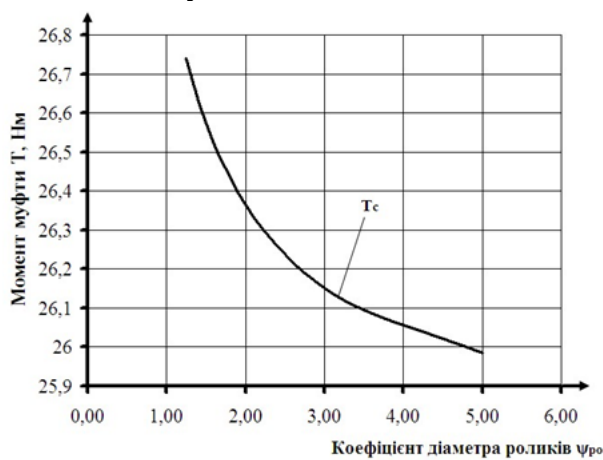
Рис. 7. Залежність моменту спрацьовування муфти від коефіцієнта діаметра осі ролика
