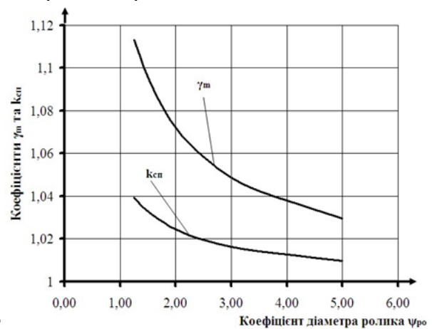
Рис. 8. Залежність коефіцієнтів точності та перевищення номінального моменту від коефіцієнта діаметра осі ролика
