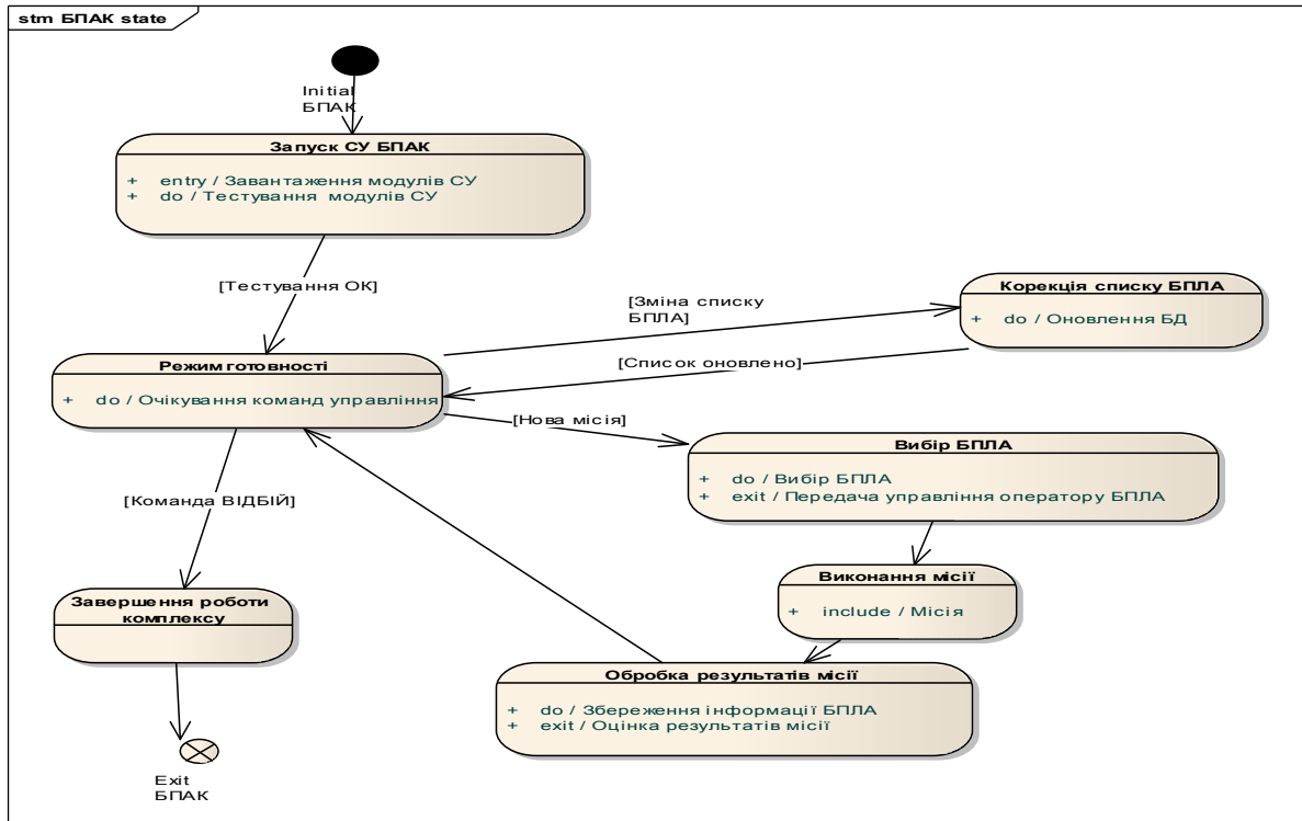
Рис. 3. Діаграма станів для наземної апаратури БпАК
