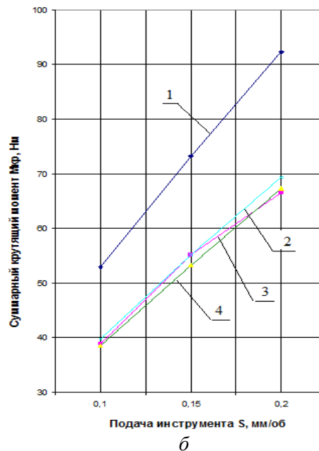
Рис. 2. Влияние подачи инструмента на: а – суммарную осевую составляющую; б – суммарный крутящий момент;
