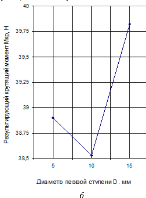
Рис. 3. Влияние величины первой ступени трехступенчатого сверла на: а – суммарную осевую силу резания; б – суммарный крутящий момент;
