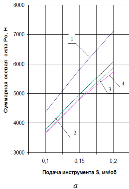
Рис. 2. Влияние подачи инструмента на: а – суммарную осевую составляющую; б – суммарный крутящий момент;
