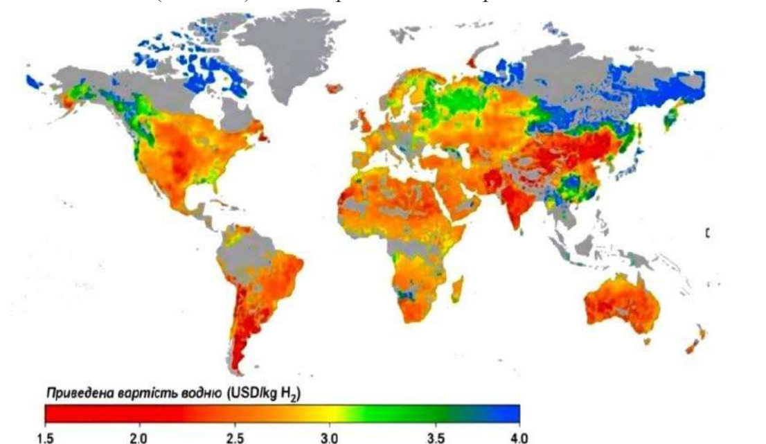
Рис. 1. Картосхема потенціалу сонячної і вітрової енергії у світі з приведеною вартістю виробництва чистого водню [16; 17; 21]
