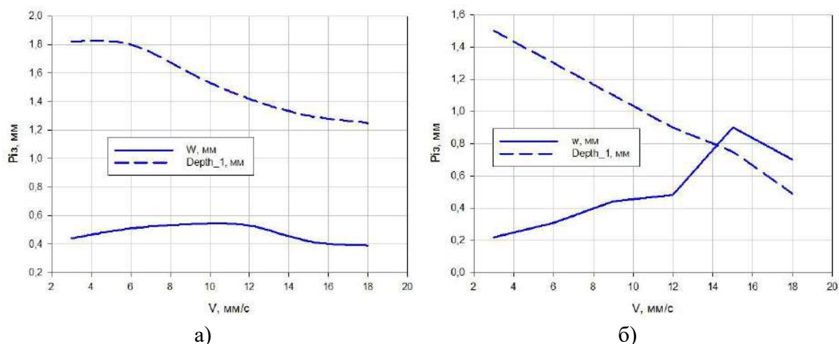
Рис. 2. Залежності глибини depth\_1 та ширини W лазерного різь КНБ від швидкості обробки, кількість проходів n=8 , частота слідування імпульсів f=15 Гц при різних значеннях тиску робочого газу: а)- P=0,4 Атм.; б)- P=2 Атм.
