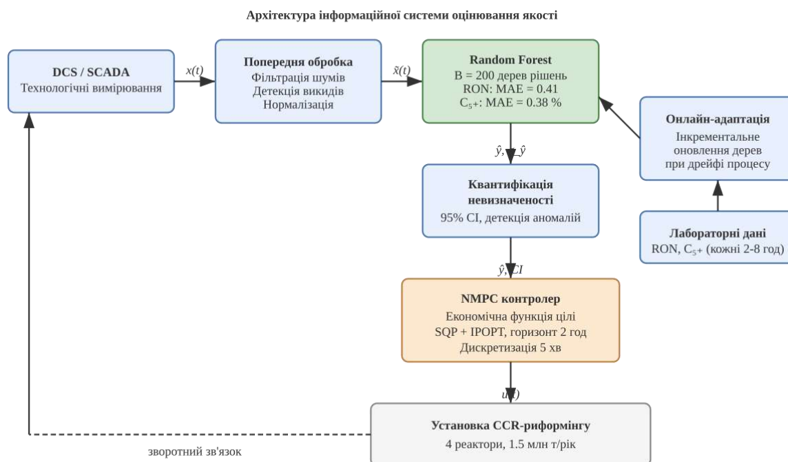
Рис. 1. Архітектура інформаційної системи оцінювання якості
