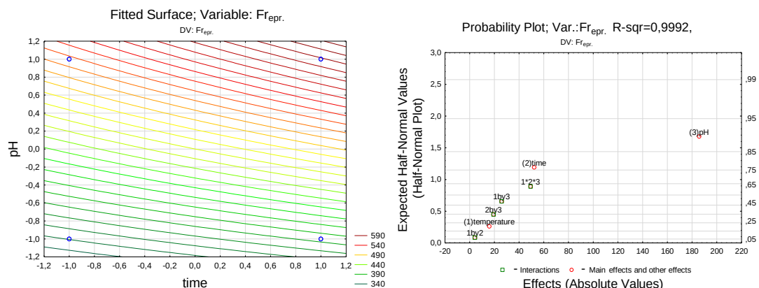
Рис. 4 Графіки залежності резонансного поля на ЕПР спектрі від параметрів синтезу a - H_r = f(t, \tau) ; b - H_r = f(pH, t) ; c - H_r = f(pH, \tau) ; d - графік вірогідності значень
