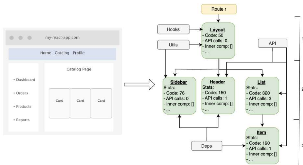
Рис. 1. Графічне представлення графа компонентів та маршрутів, що представляє структуру вебдодатка
