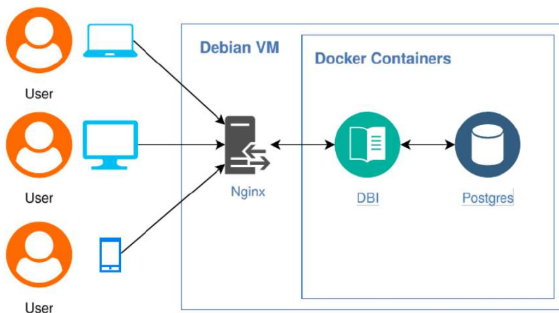
Рис. 2. Узагальнена архітектура системи каталогізації книжкових метаданих
