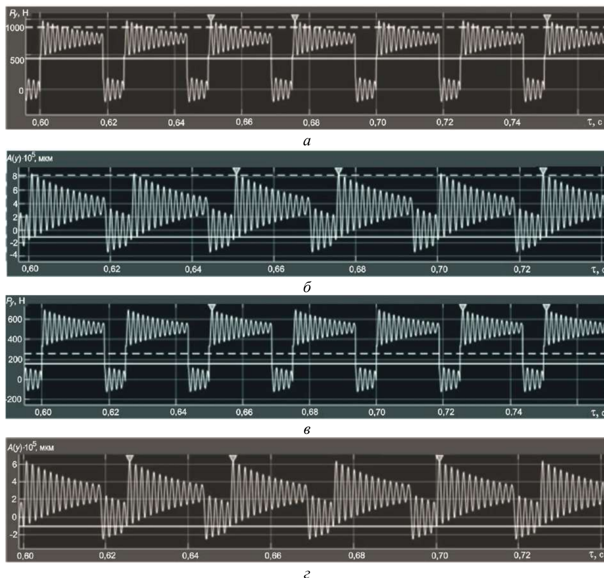
Рис. 6. Зміна сили P_y (а, в) та амплітуди вібропереміщень A(y) різця (б, г) при обробці косокутним інструментом з прямолінійною різальною кромкою: а, б – \lambda = 30^\circ ; в, г – \lambda = 60^\circ
