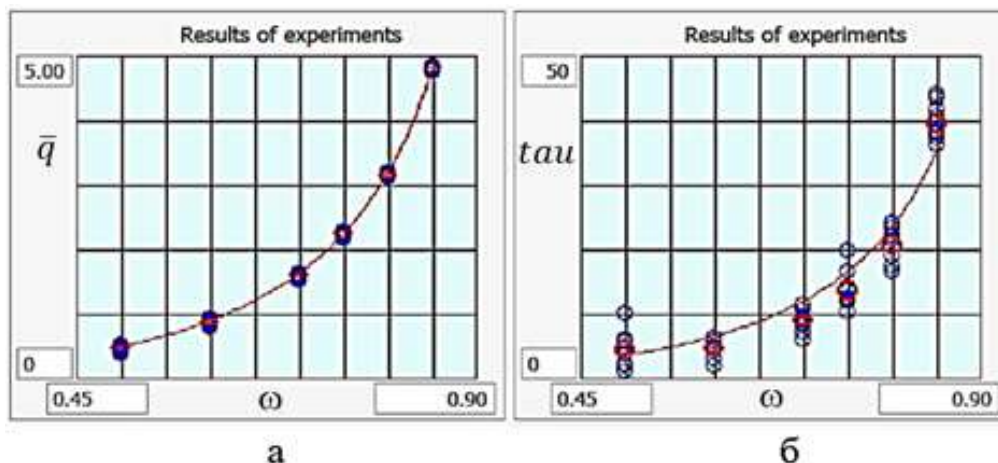
Рис. 4. Залежність параметрів СМО від коефіцієнта завантаження:
