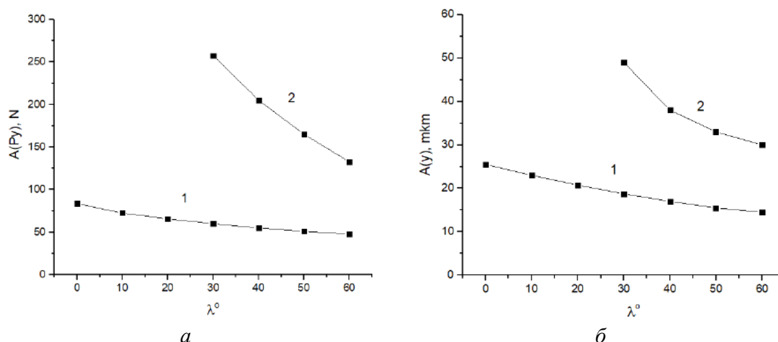
Рис. 7. Вплив кута нахилу різальної кромки \lambda на максимальну амплітуду сили різання A(P_{y\max}) (а) та амплітуду вібропереміщень A(y) (б) для інструменту з радіусною різальною кромкою (1) та косокутного інструменту з прямолінійною різальною кромкою (2)
