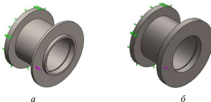
Рис. 8. Схема закріплення та прикладання осьової сили різання:
