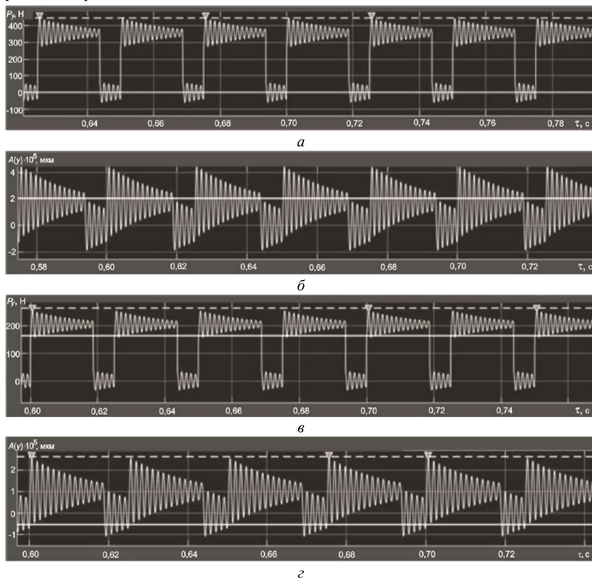
Рис. 5. Зміна сили P_y (а, в) та амплітуди вібропереміщень A(y) різця (б, г) при обробці інструментами з радіусною різальною кромкою: \lambda = 0^\circ (а, б); \lambda = 60^\circ (в, г)
