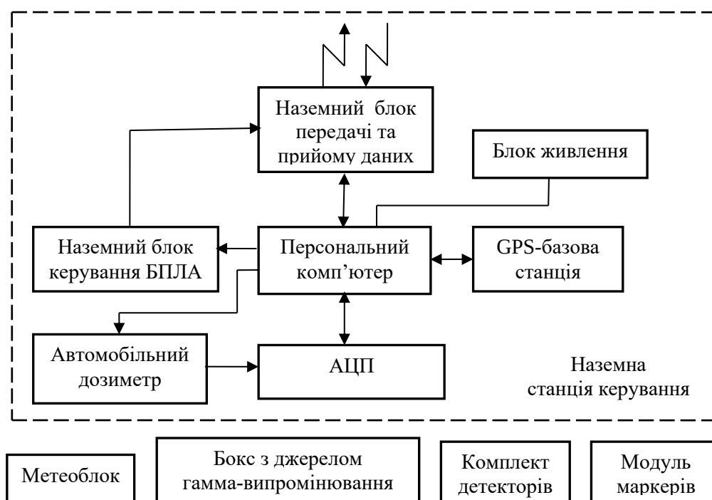
Рис. 3. Блок-схема обладнання СКТРЗ на наземному транспортному засобі [25]
