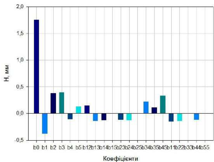
Рис. 1. Рангові діаграми коефіцієнтів рівняння регресії, які описують процес лазерного різання кубічного нітриду бору: а – ширина різу; б – глибина різу; в – глибина перфорації
