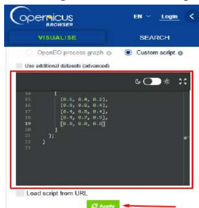
Рис. 15. Поле введення користувацького коду для розрахунку NDWI
