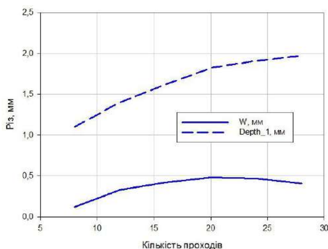
Рис. 4. Залежності глибини та ширини лазерного різку від кількості проходів сфокусованого лазерного випромінювання ( V=16 мм/с, f=25 Гц, P=2 Атм)
