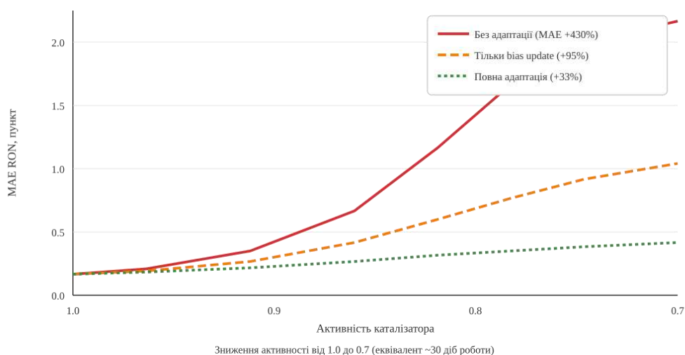
Рис. 3. Ефективність адаптації при дезактивації каталізатора
