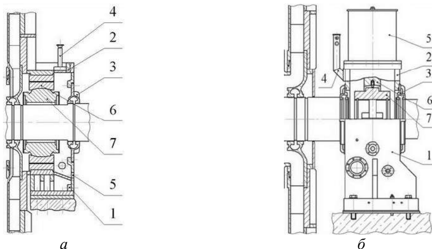
Рис. 1. Склад вальниці важкого турбогенератора:
