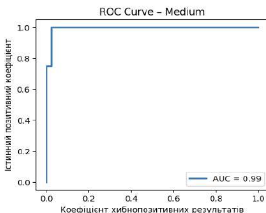
Рис. 4. ROC-крива для класу Medium
