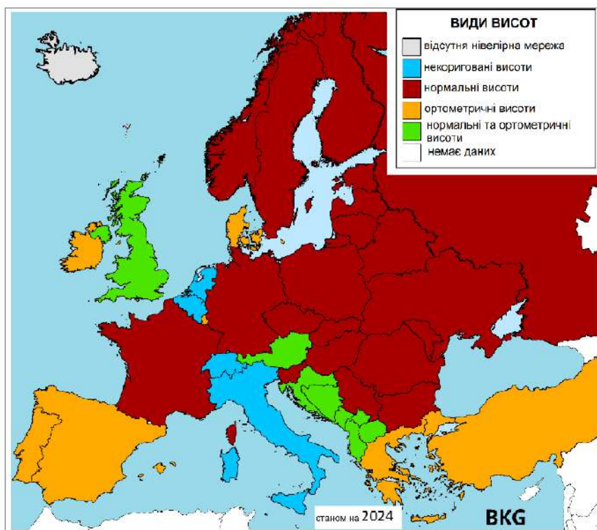
Рис. 2. Види висот національних систем висот країн Європи
