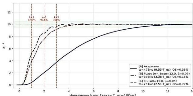
Рис. 3. Перехідний процес фаззі-регулятора, ступінчаста зміна 0^\circ - 10^\circ
