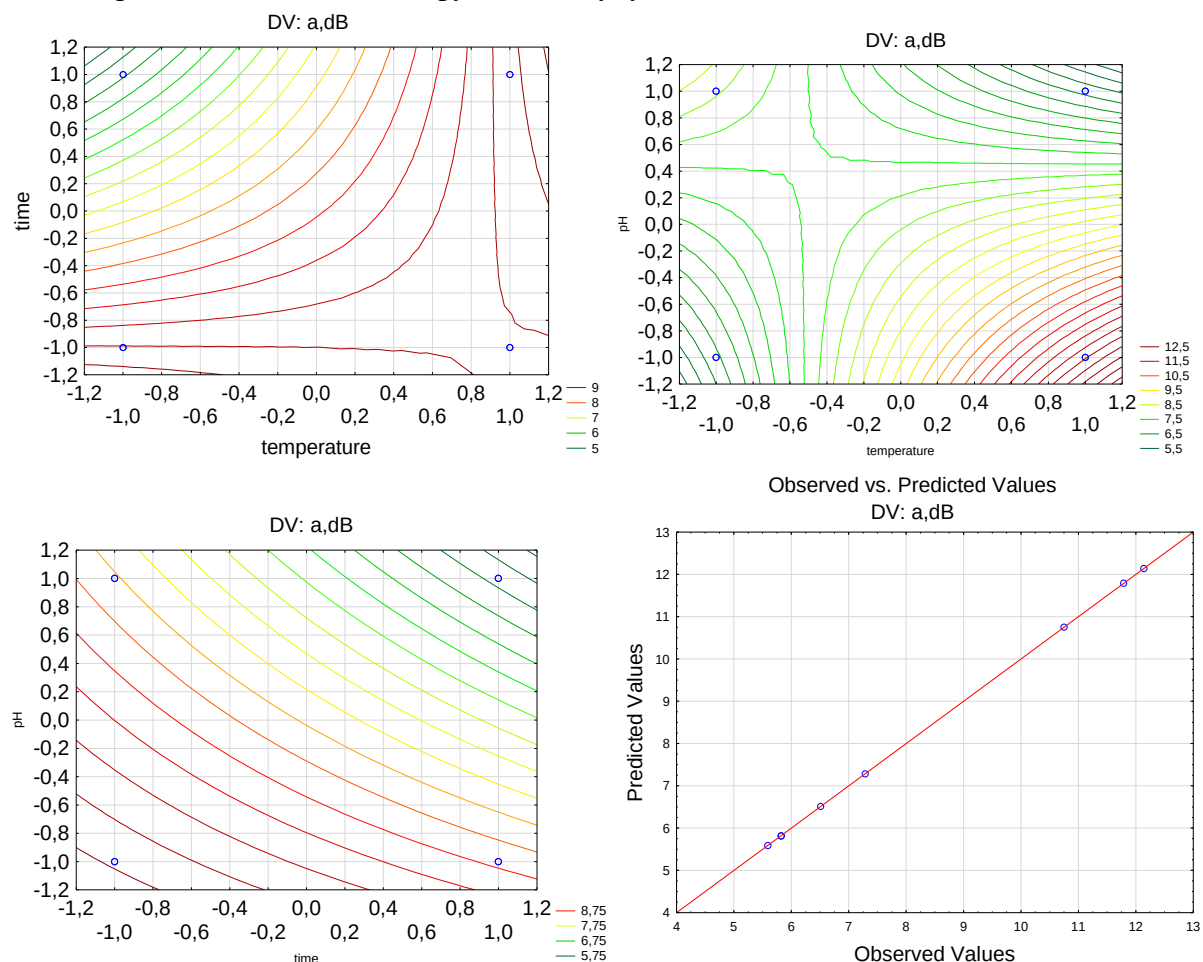
Рис. 2 Графіки залежності поглинання електромагнітного випромінювання від параметрів синтезу а-- a=f(t, \tau) б-- a=f(\text{pH}, t) в-- a=f(\text{pH}, \tau) , г - спостережувані та прогнозовані значення
