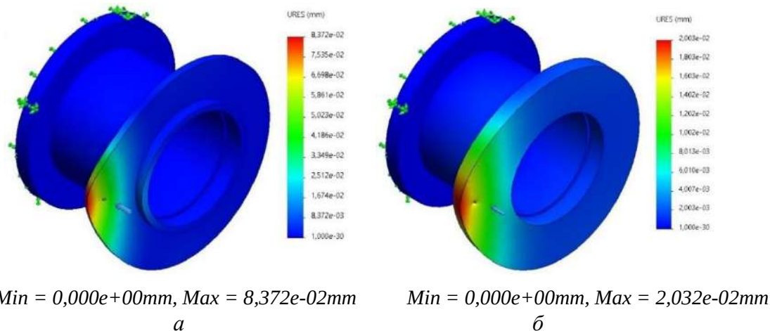
Рис. 9. Переміщення заготовки під дією сили різання при свердлінні:
