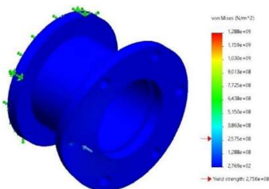
Рис. 15. Розподіл напружень (Von Mises Stress) при обробці останнього отвору
