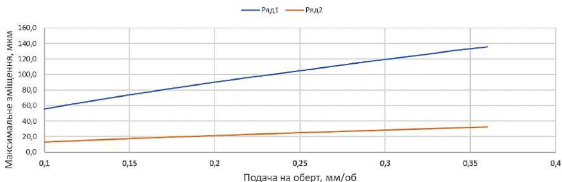
Рис. 12. Графік максимального переміщення деталі залежно від подачі на оберт Джерело: розроблено авторами.
