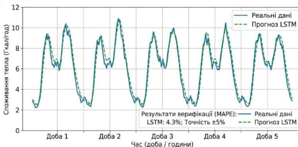
Рис. 3. Порівняння реальних та прогнозних даних споживання тепла на моделі LSTM Джерело: отримано авторами.
